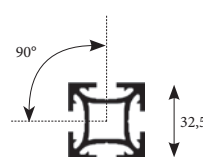
Mât 4 départs
