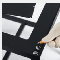
Fixation du piètement sur le cadre supérieur, recouvert par le plateau de la vitrine
