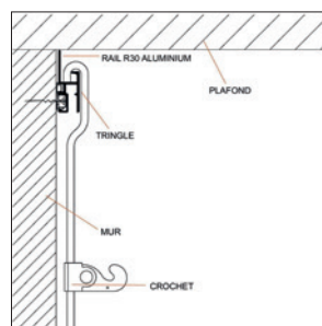
Accrochage par tige
