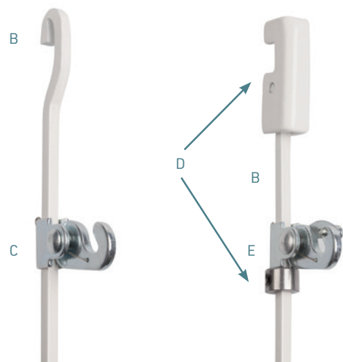
Solution Classique
