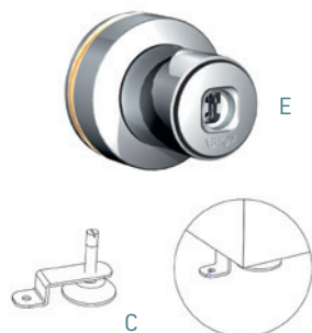
Verrouillage au sol de la vitrine RAL 9005 ou RAL 9016
